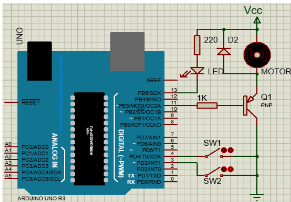
Hình 1: Mạch arduino điều khiển động cơ và Led
